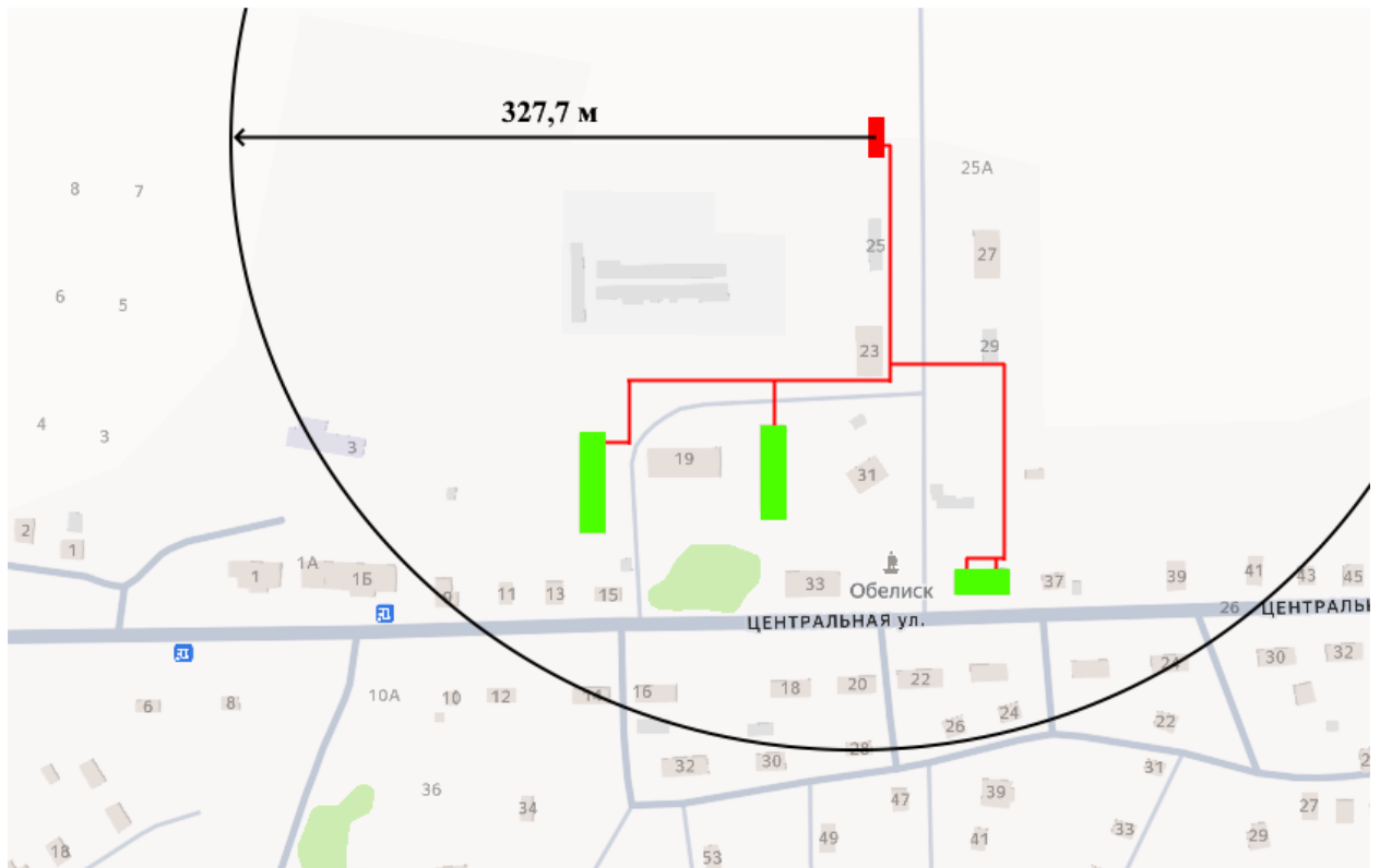
Рисунок. Радиус эффективного теплоснабжения дер. Коротиха
